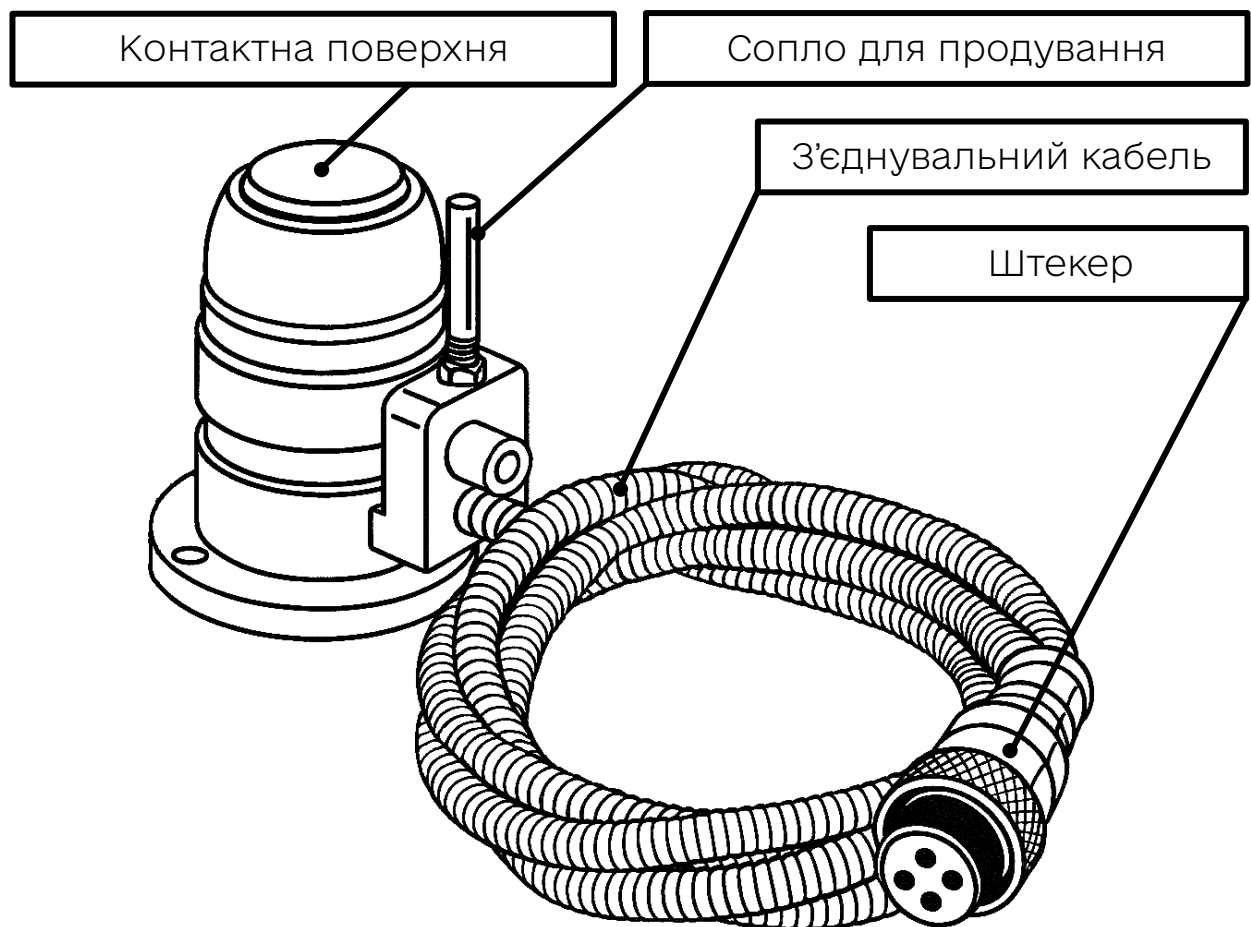
Рис. 2.2 Загальний вигляд типового контактного датчика
